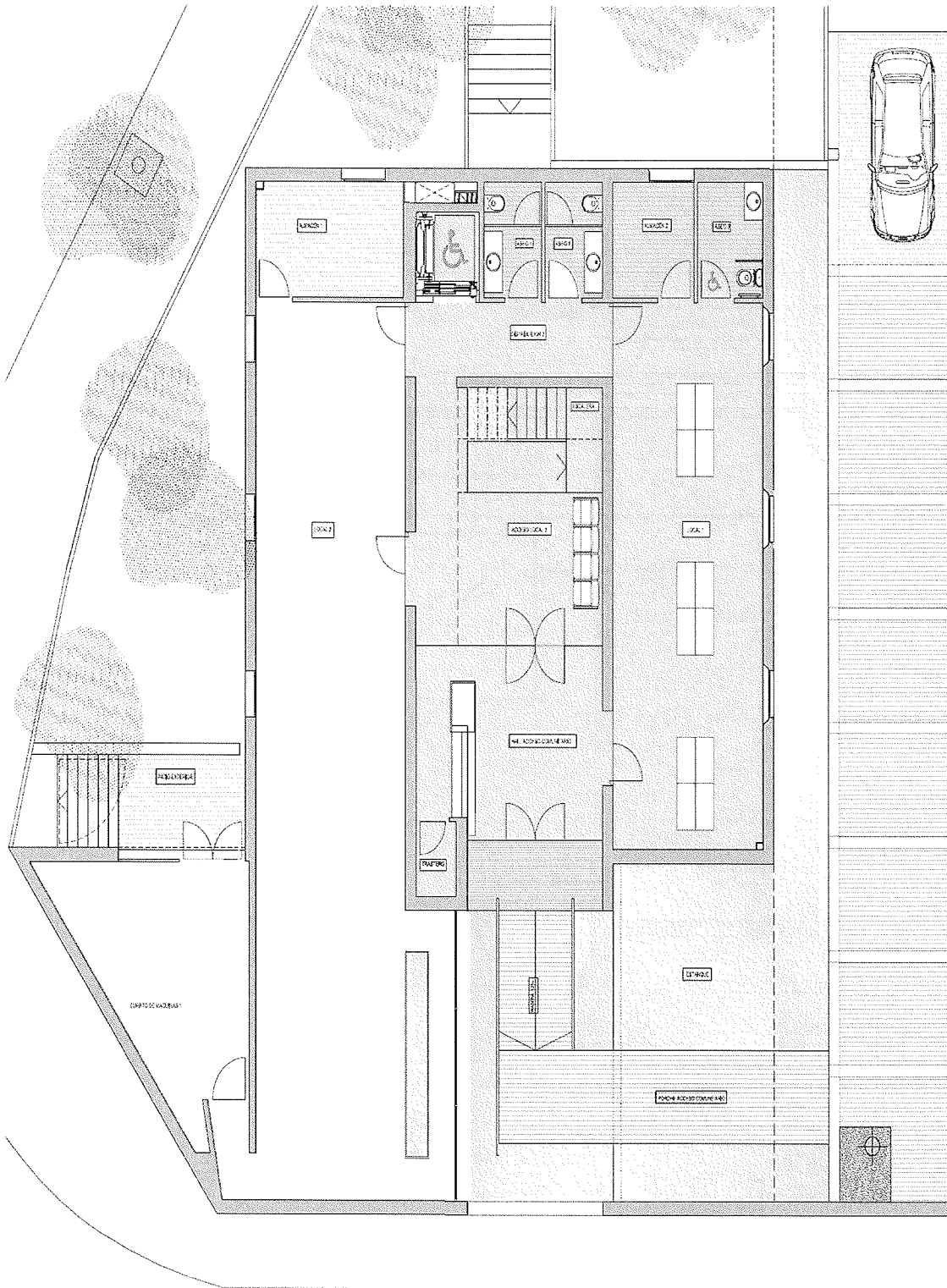
PLANTA SEMISOTANO E: 1/50
